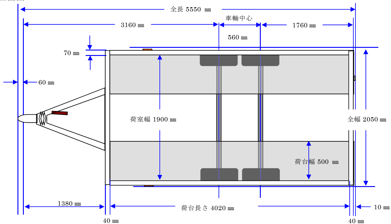
○上面図
