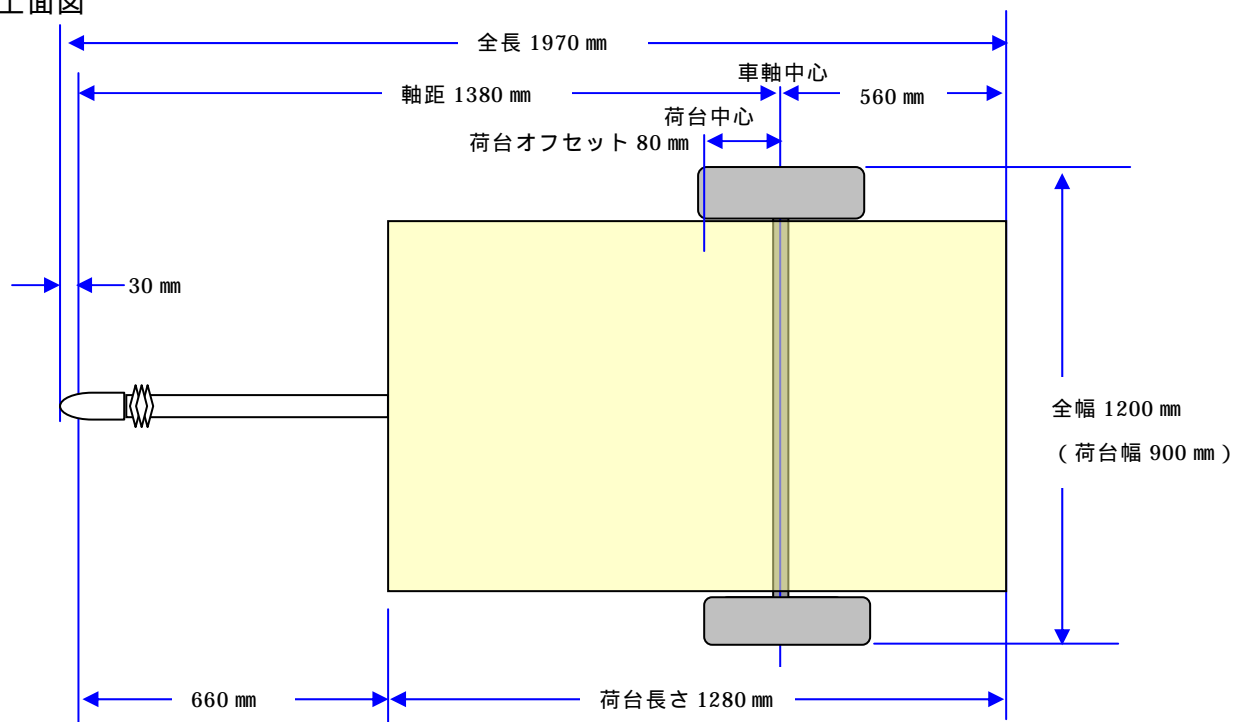
上面図
